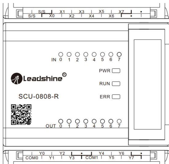
图 5-5 SCU-0808-R模块端子丝印
