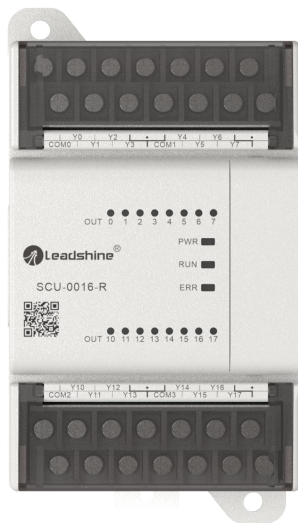
图 4-3 SCU-0016-R模块外观示意
