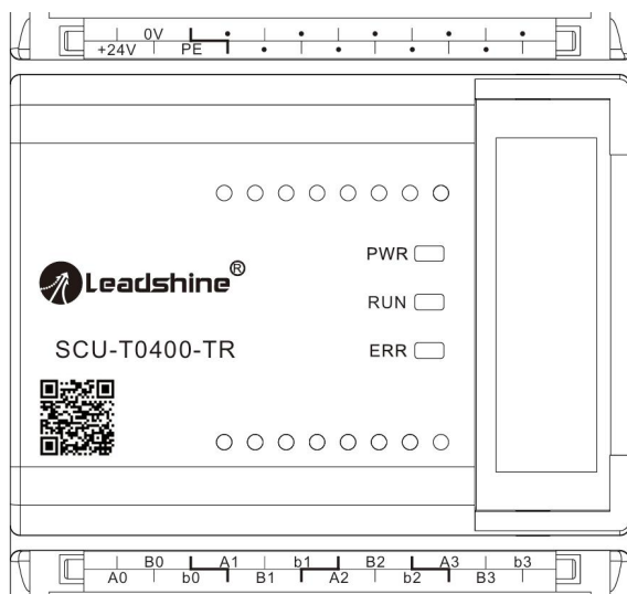
图 8-1 SCU-T0400-TR模块外观示意
