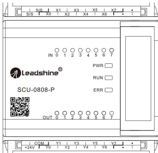
图 5-5 SCU-0808-P模块端子丝印
