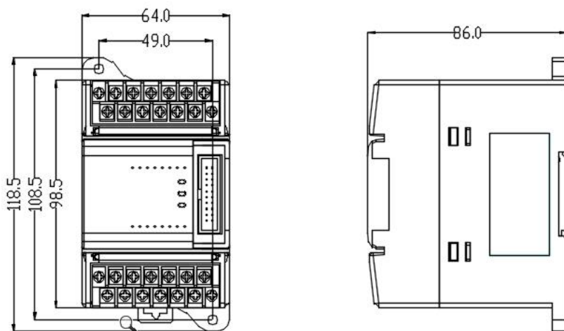
图 4-4 数字量输出模块尺寸
