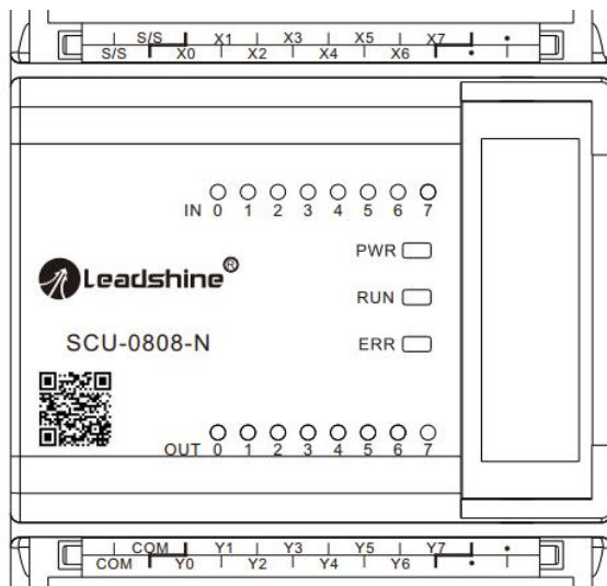
图 5-4 SCU-0808-N模块端子丝印
