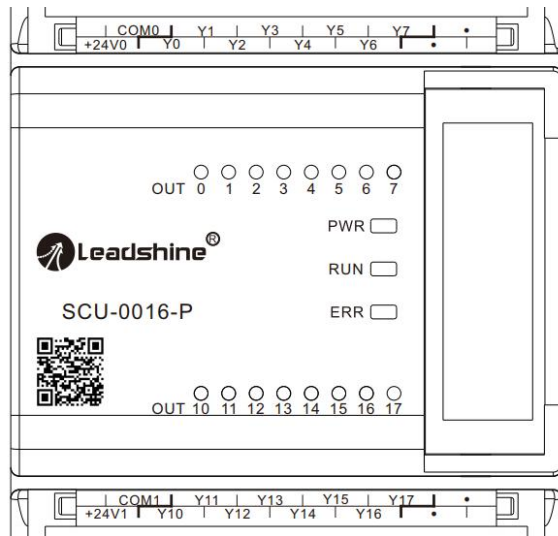
图 4-6 SCU-0016-N模块端子丝印
