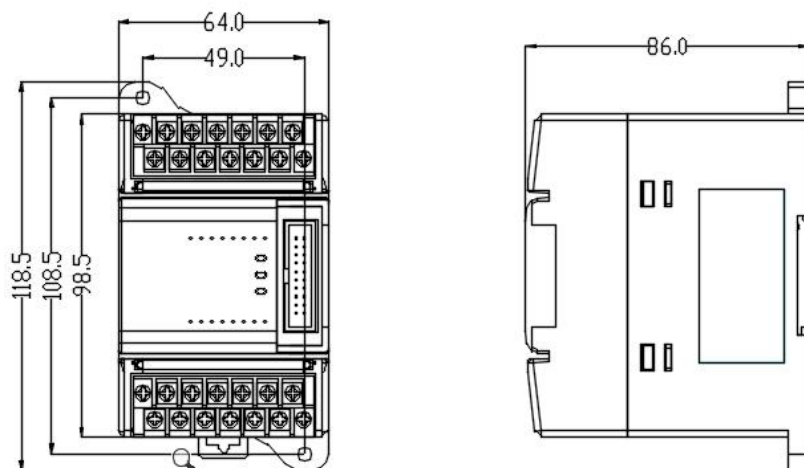
图 11-1 SCU系列扩展模块外观尺寸
