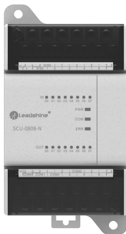
图 5-1 SCU-0808-N模块外观示意
