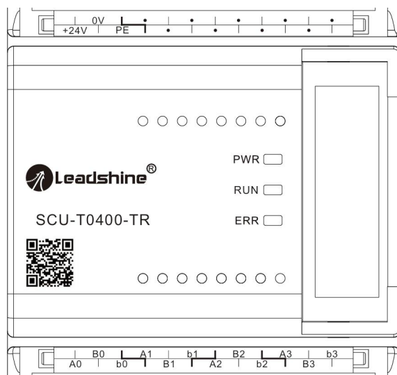
图 8-2 SCU- T0400-TR模块端子丝印
