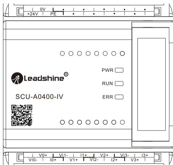
图 6-2 SCU-A0400-IV模块端子丝印
