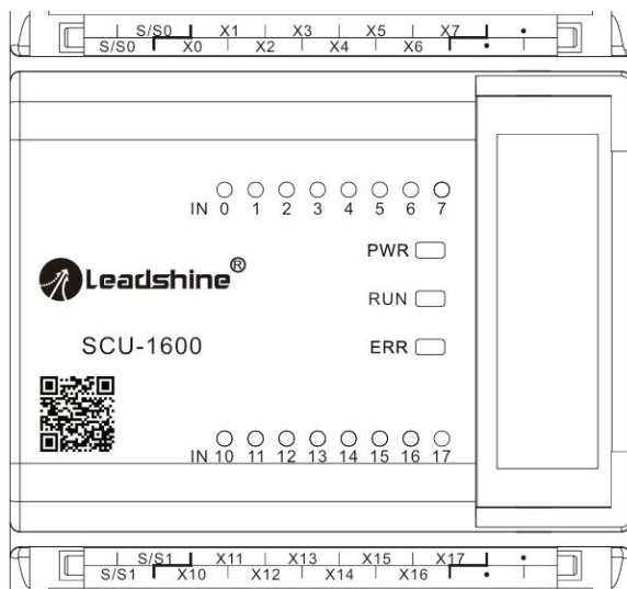
图 3-3 SCU-1600模块端子丝印
