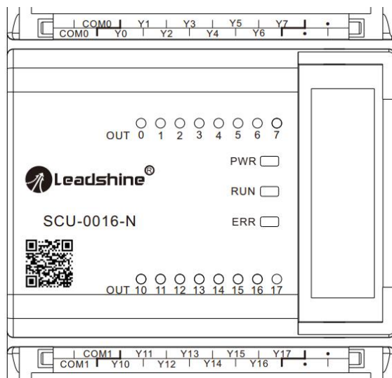
图 4-5 SCU-0016-N模块端子丝印
