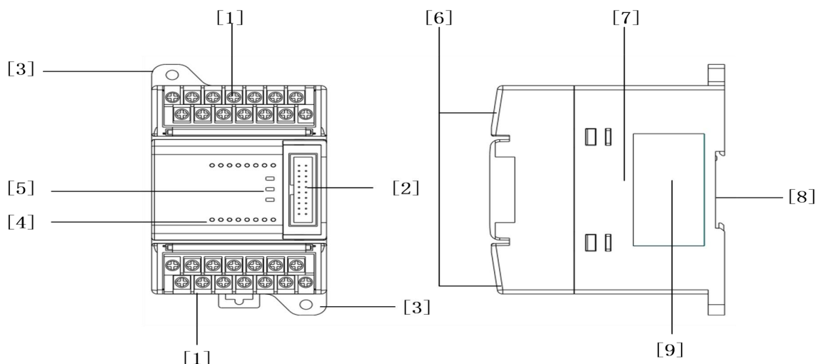
图 2-1 SCU系列产品外观定义图
