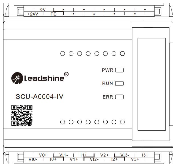
图 7-2 SCU-A0004-IV模块端子丝印
