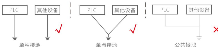
图 1-1 接地类型图
