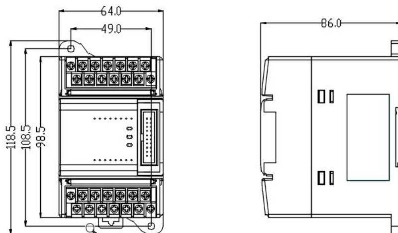
图 3-2 数字量输入模块尺寸
