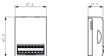
图 2-2 SCU系列扩展BD板产品正面外部接口图
