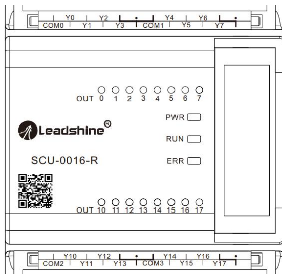
图 4-7 SCU-0016-R模块端子丝印
