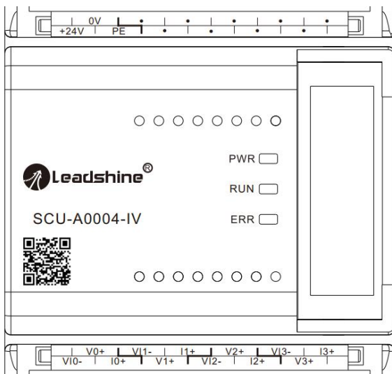
图 7-1 SCU-A0004-IV模块外观示意
